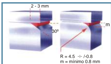
Diseño de brida con radio de acuerdo.
