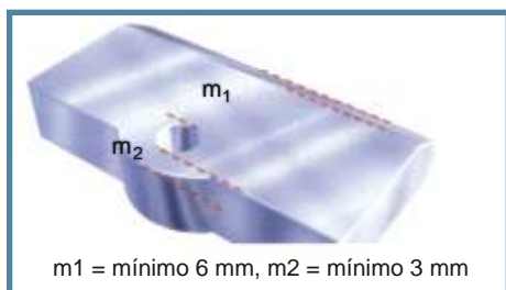
Diseño de brida con chaflán.
